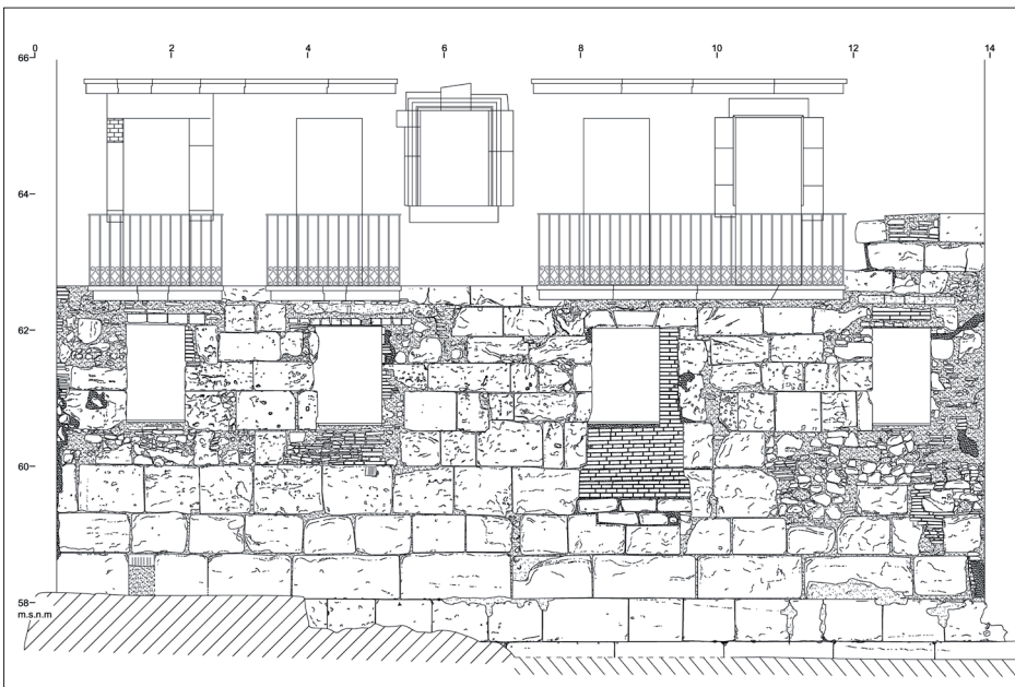
Figura 5. Alçat de la planta baixa que inclou les filades inferiors actualment ocultes sota el carrer.
