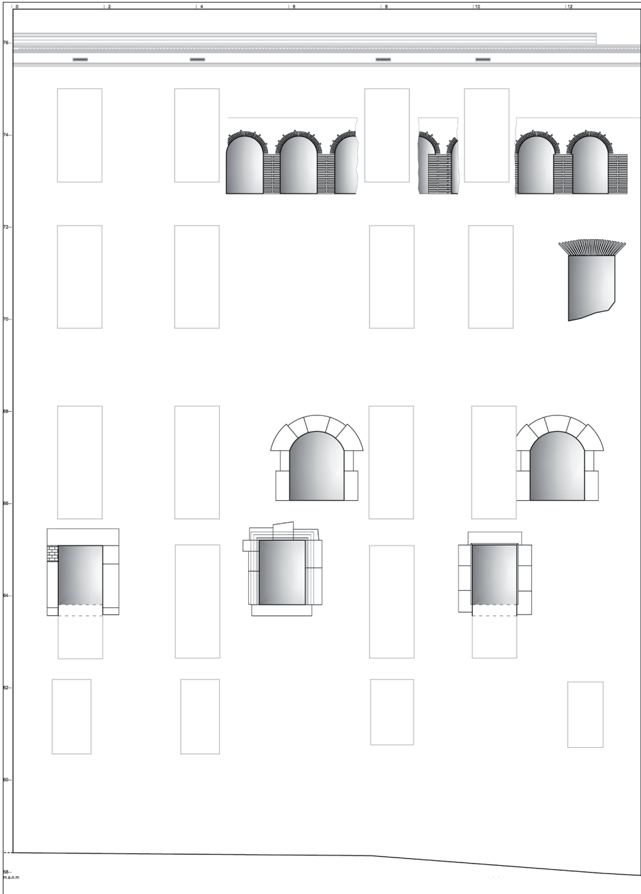
Figura 1. Alçat de la façana amb indicació de les antigues obertures (ombrejades) i indicació de les obertures actuals (en traç fi).
