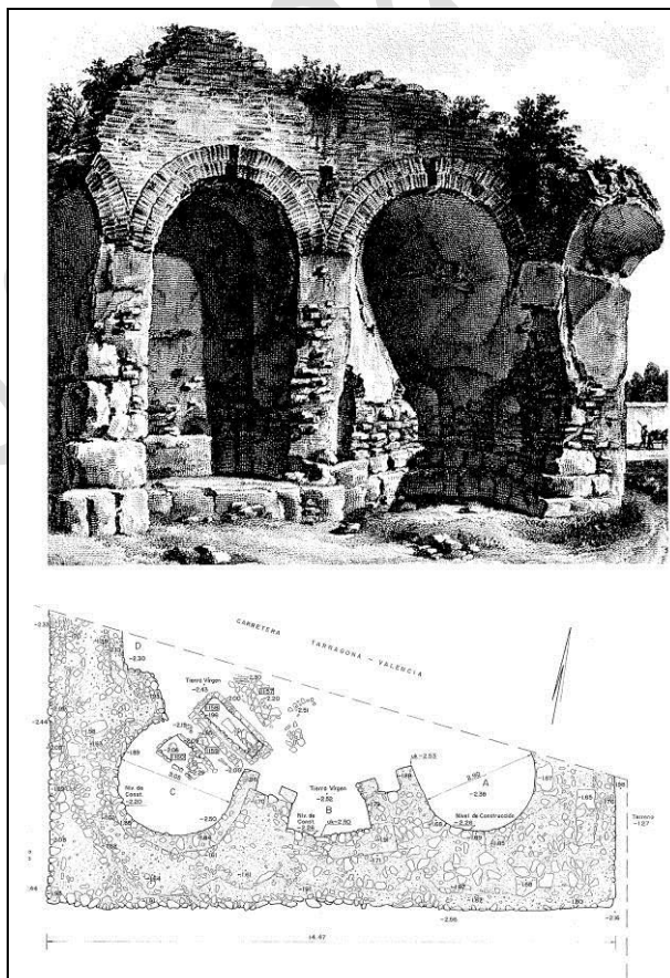
Fig. 4 Gran mausoleu de planta central de la necròpolis. Gravats d'Alexandre de Laborde a principis del segle XIX i planta de les restes conservades actualment (Th. Hauschild)
