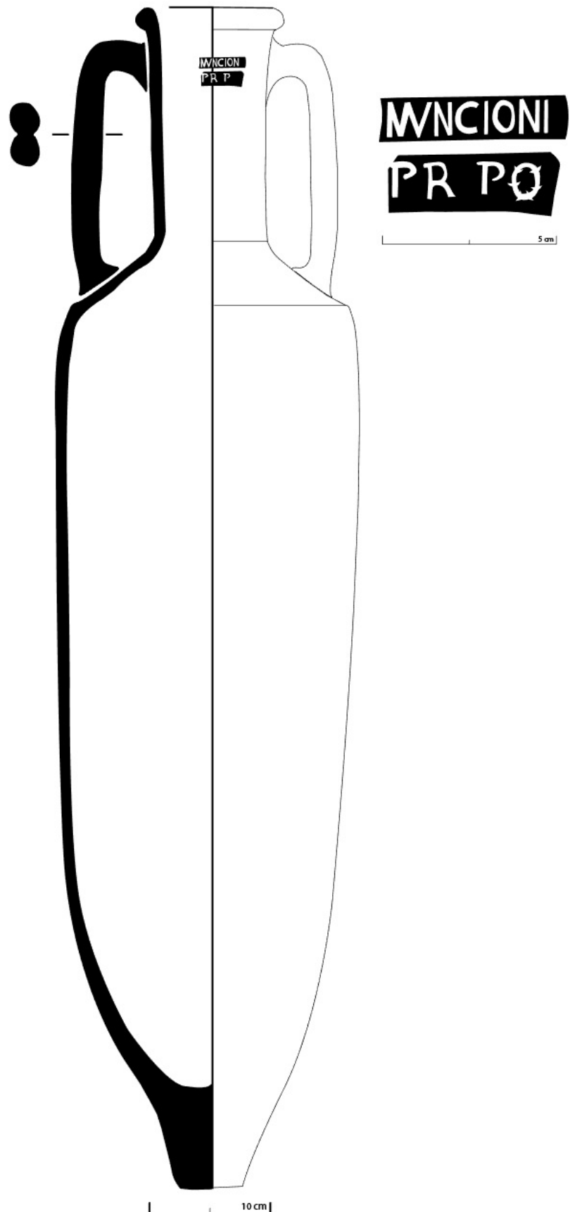
▲ Figura 1. Dibujo de la pieza (autor: Enric Colom).
